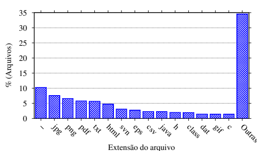
Figura 6. Distribuição da quantidade de arquivos de acordo com a extensão.
