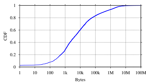
Figura 4. Distribuição do tamanho dos arquivos.
