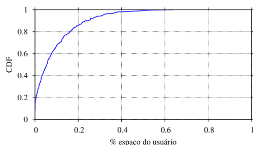
Figura 7. Dist. do consumo de espaço pelas réplicas Dropbox.
