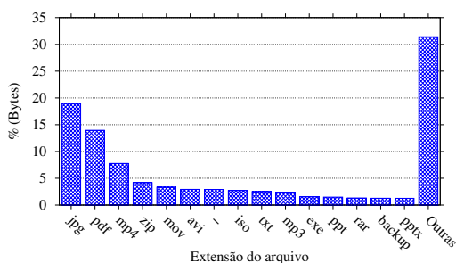
Figura 5. Distribuição do espaço ocupado de acordo com a extensão dos arquivos.
