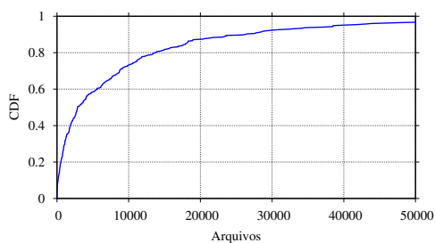
Figura 3. Distribuição do número de arquivos por usuário.
