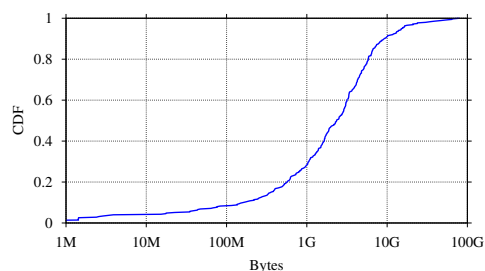
Figura 2. Distribuição do espaço ocupado por usuário.
