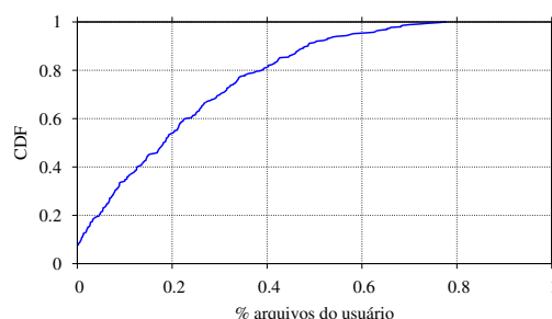
Figura 8. Dist. da quantidade de arquivos replicados.
